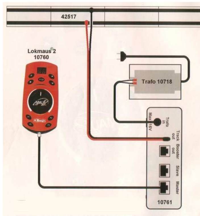
Fig. 1 – Comment brancher le coffret de départ
