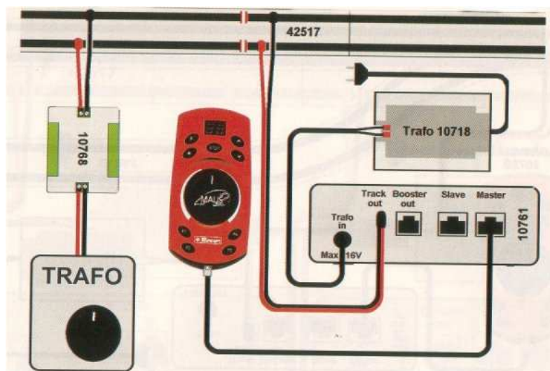
Fig. 6 – Combinaison du courant continu avec le système numérique Par le module d’interconnexion 10768
