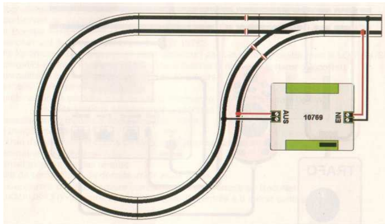
Fig. 5 – branchement d’une boucle de retournement numérique Controlée par le module 10769
