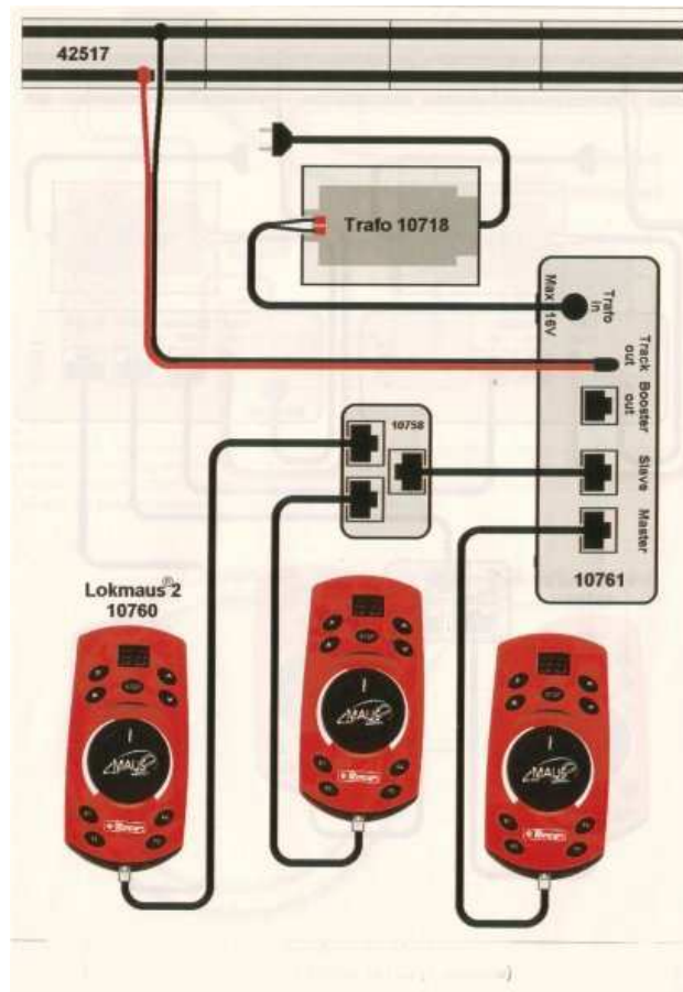
Fig. 2 – Comment brancher deux ou plusieurs LOKMAUS®2 En utilisant la fiche 10755
