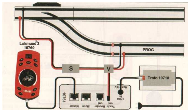
Fig. 4 – Un rail de programmation : Un interrupteur interrompt l'alimentation de la section de circulation
