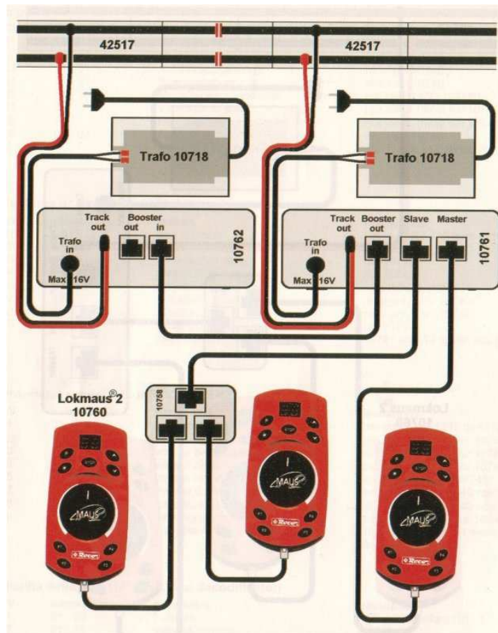
Fig. 3 - Comment brancher le booster 10762 à l'amplificateur 10761 et aux rails
