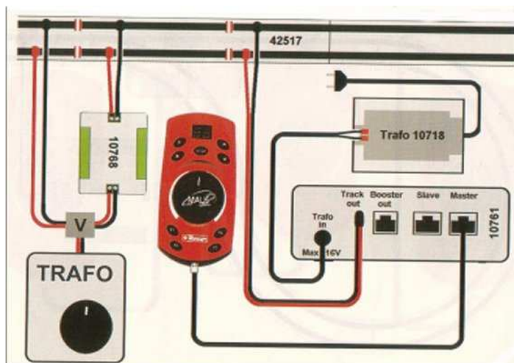
Fig. 7 – Un tronçon de transmission du système numérique au système courant continu avec le module 10768
